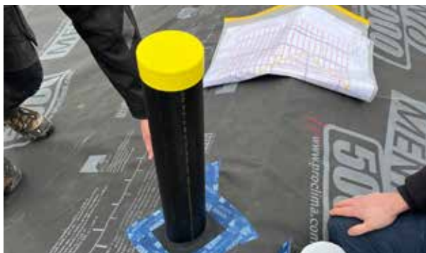
...en van een ontluuchtingspijp met ROFLEX voor \varnothing 100 -120 mm
